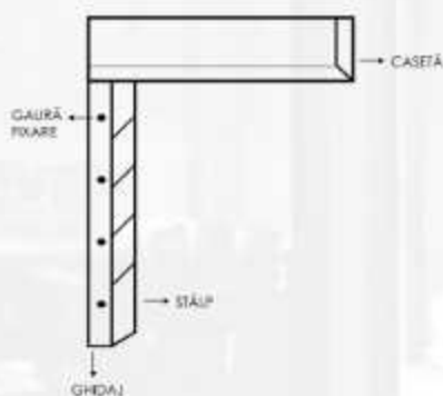
SCHITA 1. Montaj rulo cu casetă
