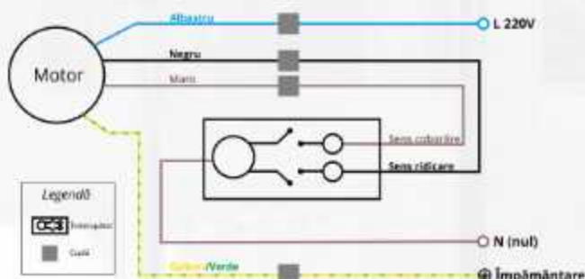
SCHITA 2. Motor cu întrerupător
